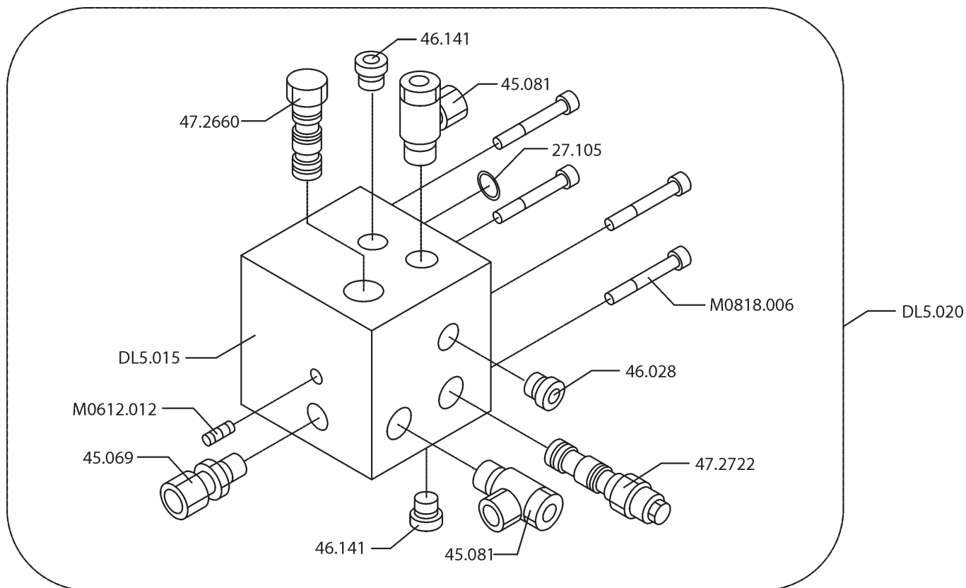
TELESKOOPPISYLINTERI -VENTTIILIPESÄN OSAT → 1791 9VA0865
