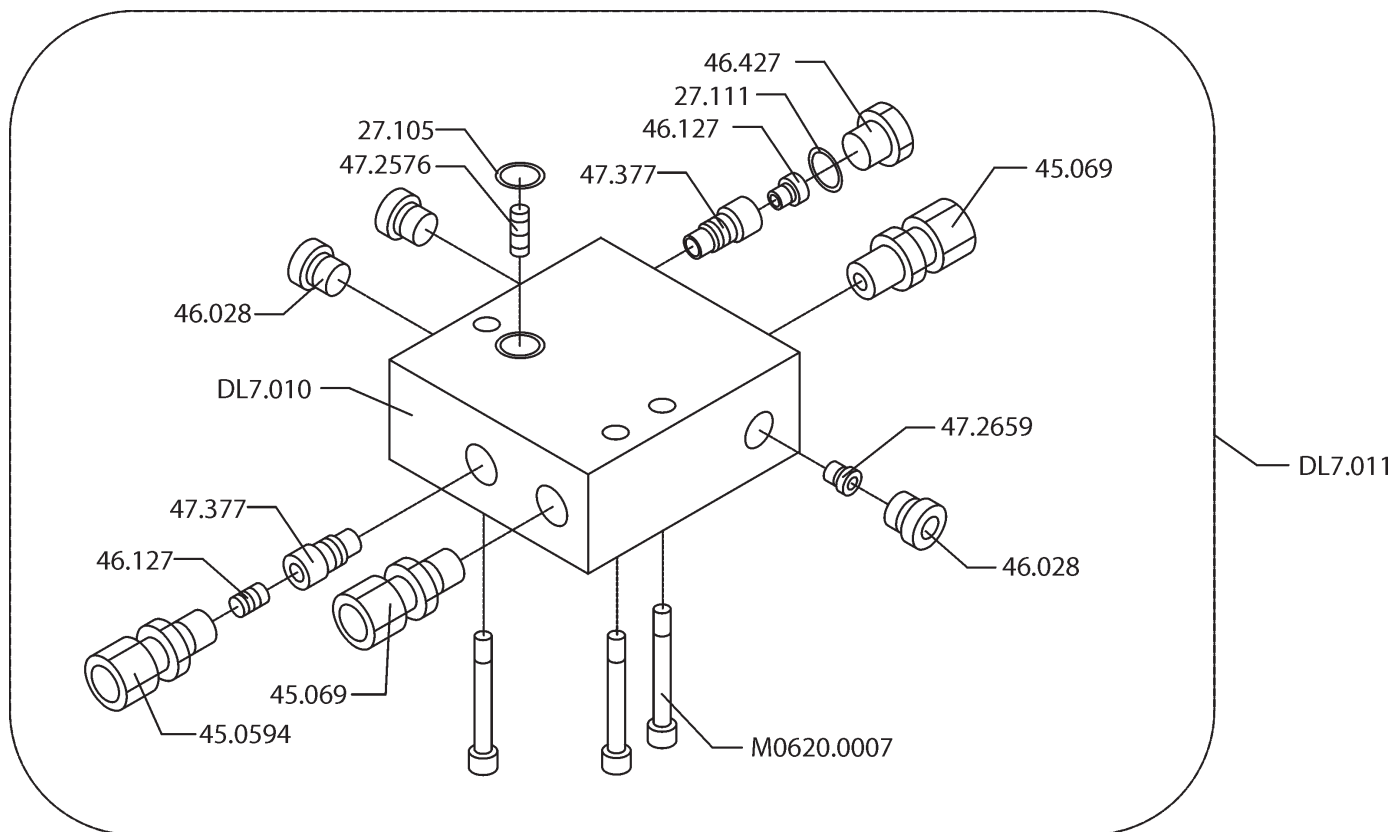
TUKIJALKASYLINTERI -VENTTIILIPESÄN OSAT → 1835 9VA1795
