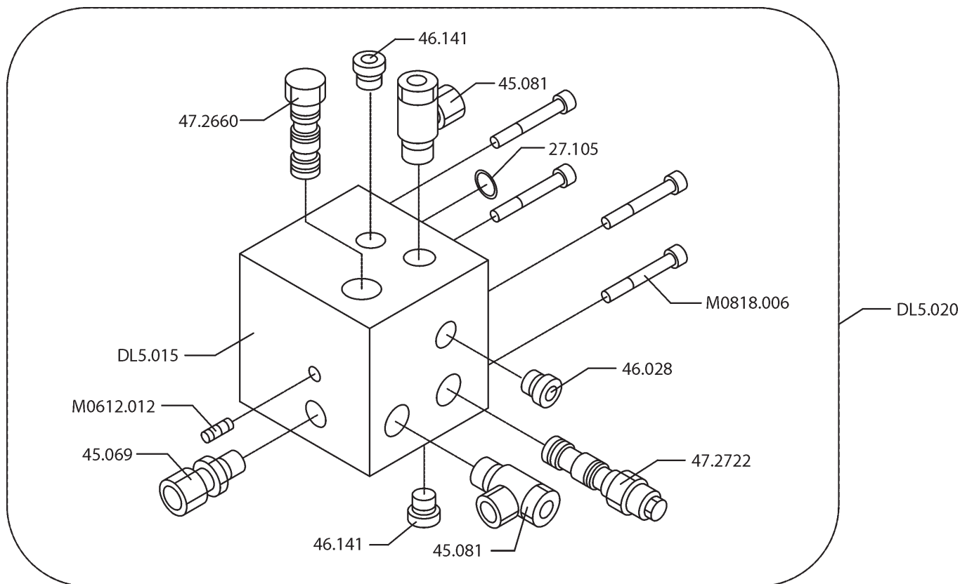
TELESKOOPPISYLINTERI -VENTTIILIPESÄN OSAT → ????? 9VA0865
