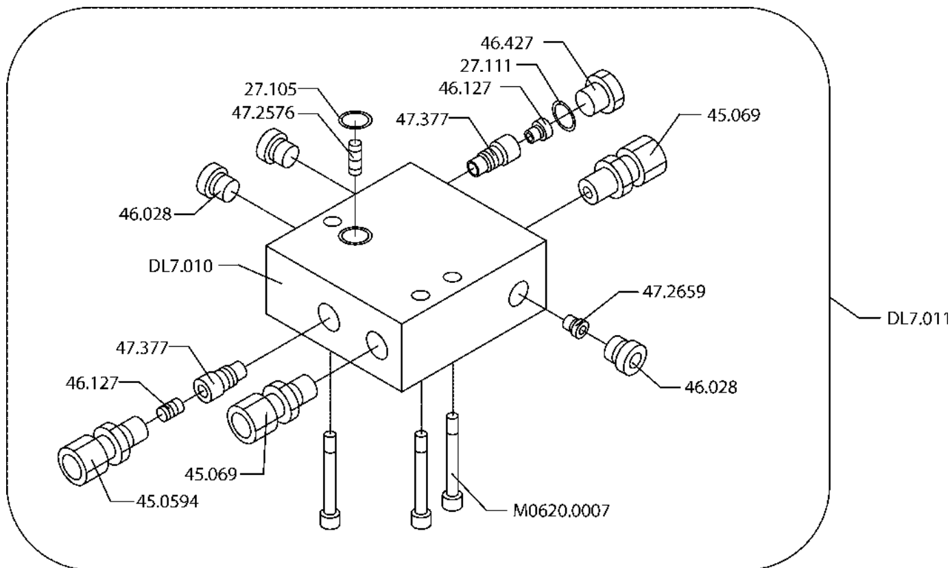
TUKIJALKASYLINTERI -VENTTIILIPESÄN OSAT → 4788 9VA1795
