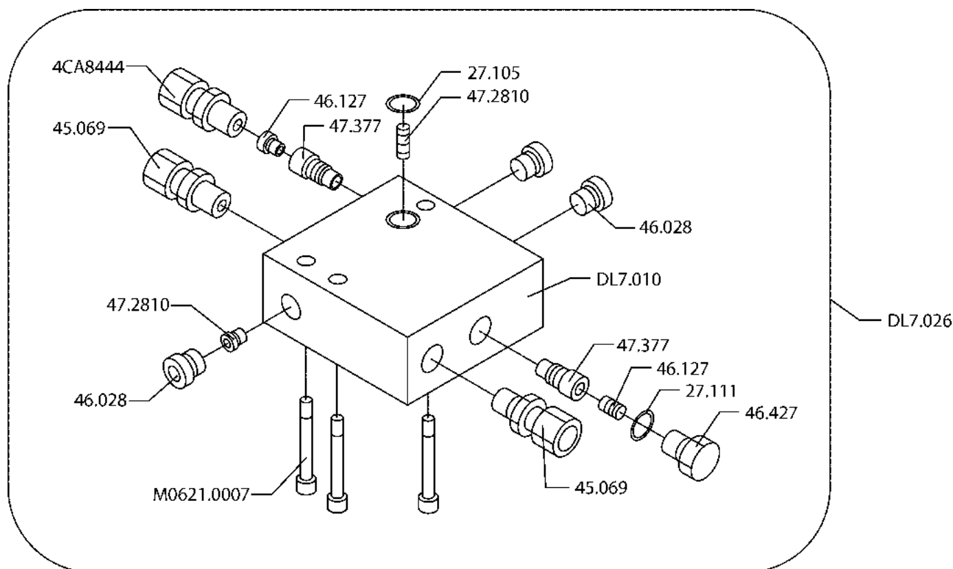
TUKIJALKASYLINTERI -VENTTIILIPESÄN OSAT → ????? 9VA1294
