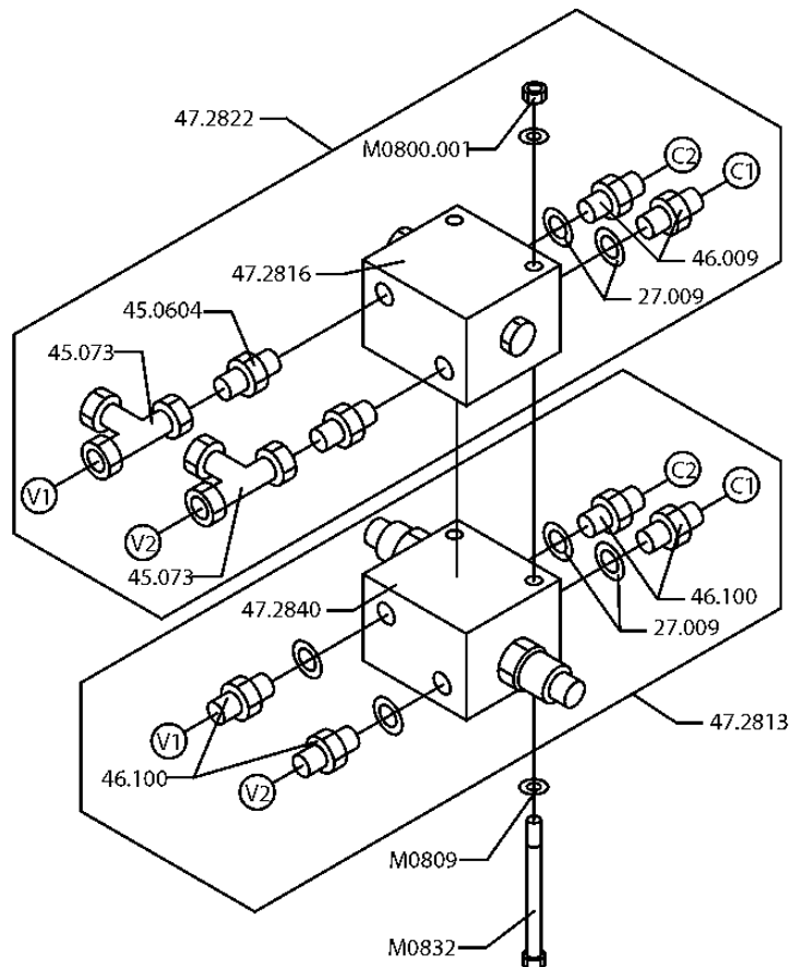
HYDRAULIIKKA, VENTTIILIT DC260XT
