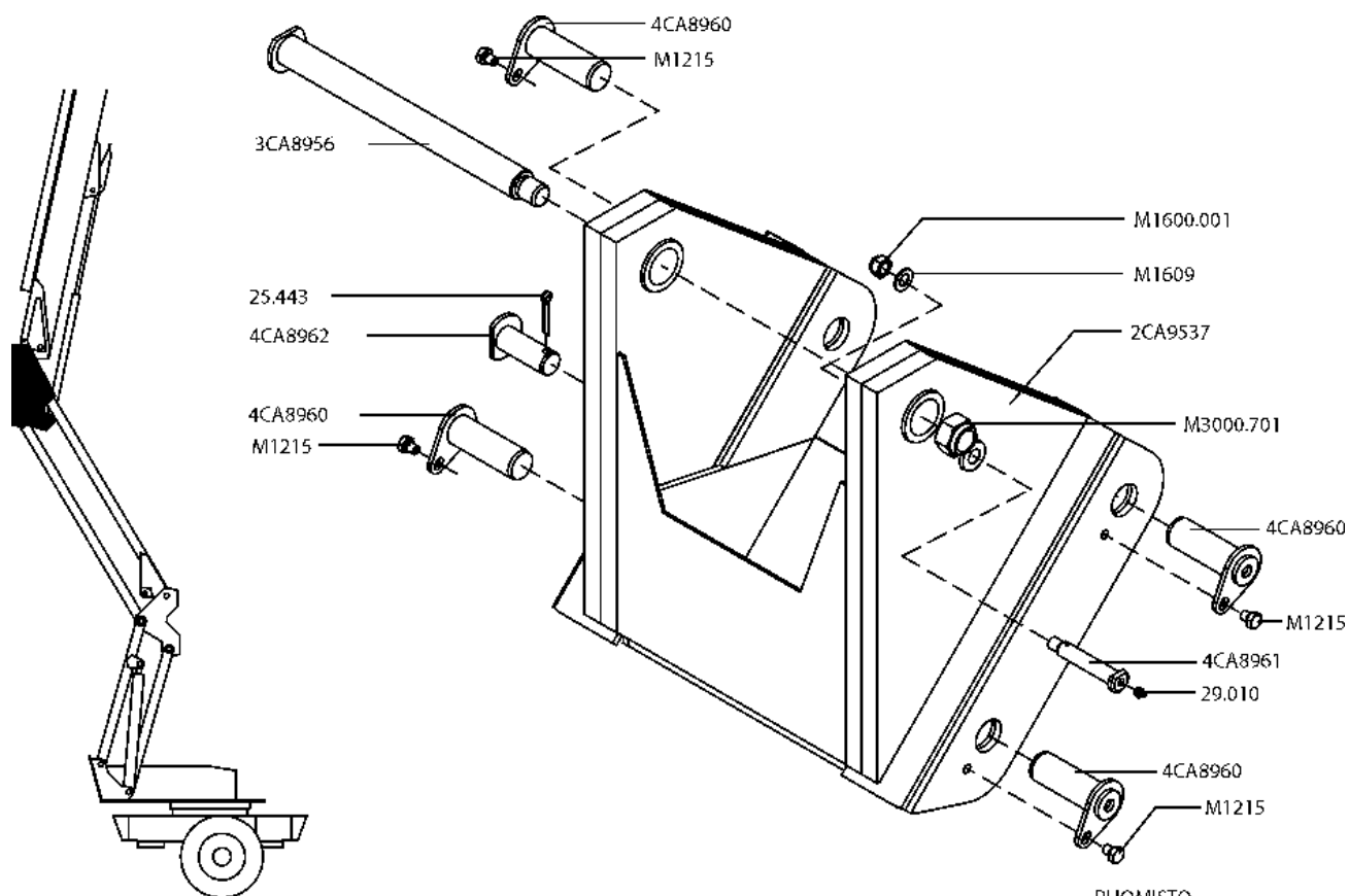
PUOMISTO -SUUNTAISVARSISTO -KIINNITYSRUNKO 26023-26177 9VA1261
