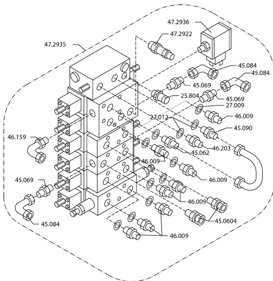
HYDRAULIIKKA -MAGNEETTIVENTTIILIT 26102-26149,26151-26154 9VA1872
