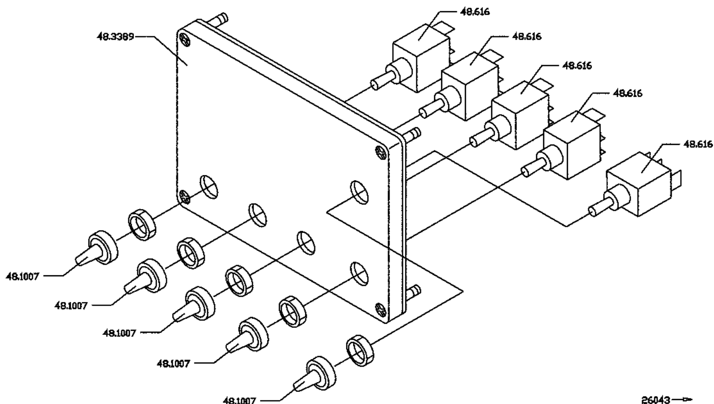
26043 → TUKIJALKAKOTELON KANSI DC260XT,DC230T 9VA1414
