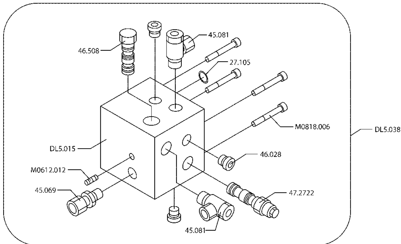
TELESKOOPPISYLINTERI -VENTTIILIPESÄN OSAT → 26174 9VA1295
