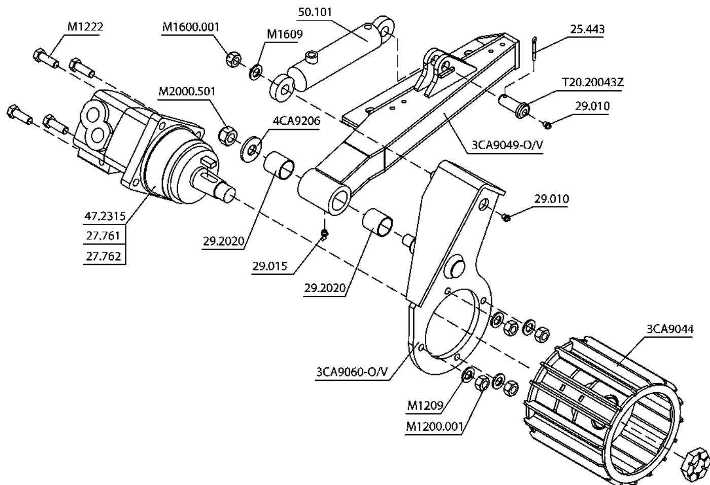
DC260XT AJOLAITE 9VA1266 26108
