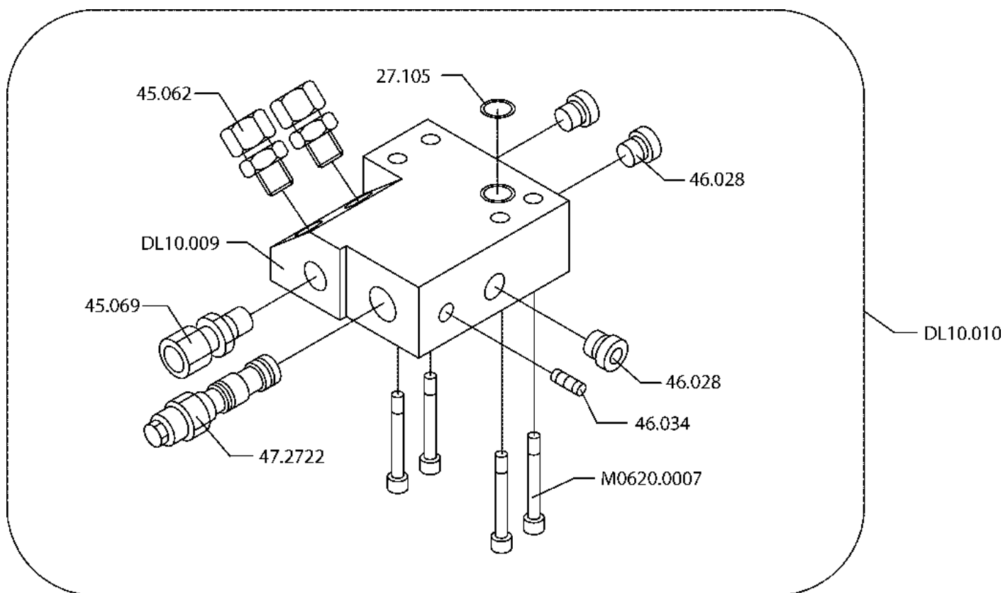
ORJASYLINTERI -VENTTIILIPESÄN OSAT → 26139 9VA0939
